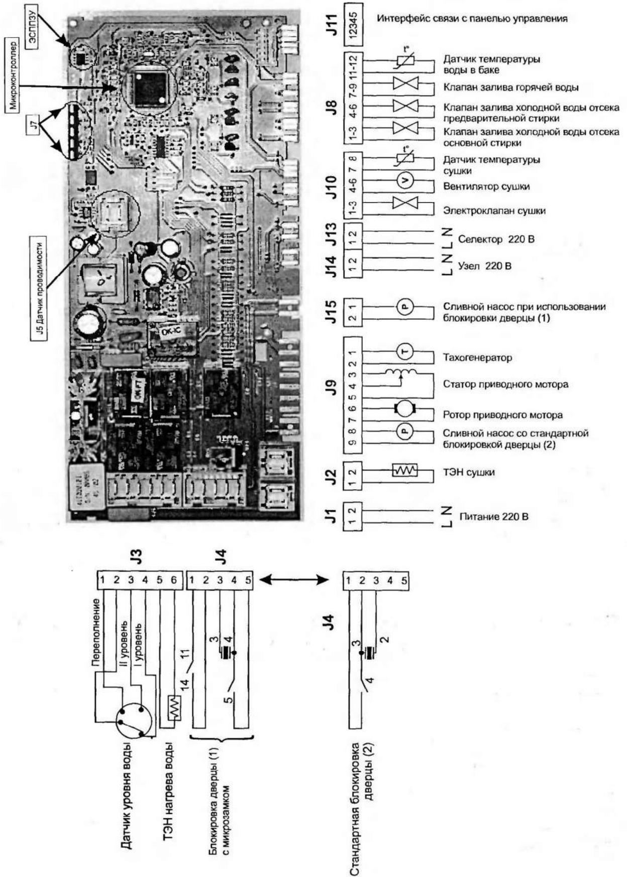
Рис. 5.2.1. Электронный модуль EVO-II и его внешние соединения
