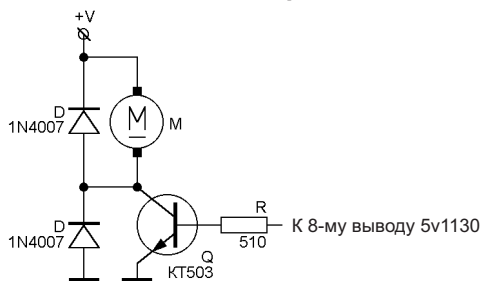
Рис.4 Подключение слаботочного коллекторного двигателя постоянного тока.
