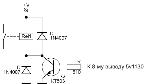
Рис.5 Подключение реле постоянного тока.
