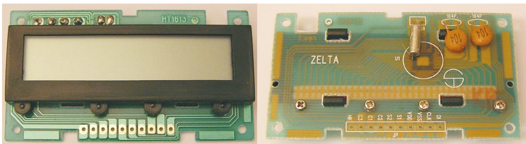
Рис.2 Внешний вид индикатора HT1613, применяемого с микроконтроллером 5v1130.
