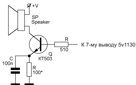
Рис.8 Подключение низкоомной динамической головки.
