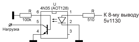
Рис.7 Подключение нагрузки с гальванической развязкой оптроном.
