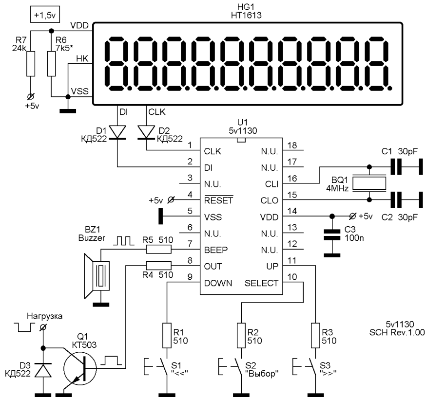
Рис.1 5v1130 Типовая принципиальная электрическая схема включения.
