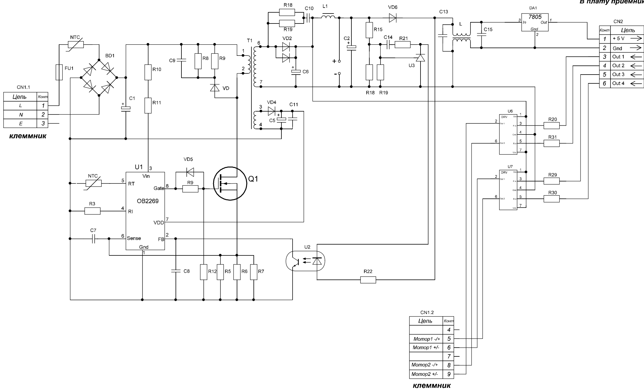
Плата питания Радиовыключателя штор
