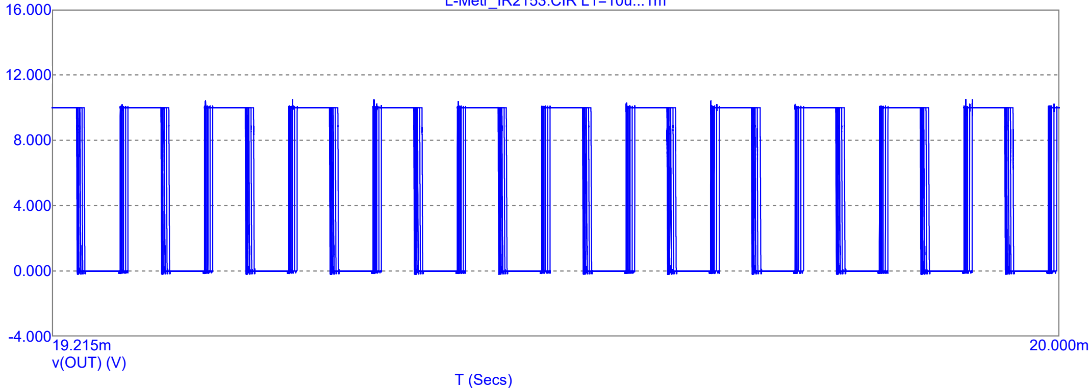
L-Metr_IR2153.CIR L1=10u...1m
