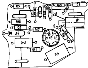
Рис. 9. Схема расположения элементов на фторопластовой плате усилителя У.
