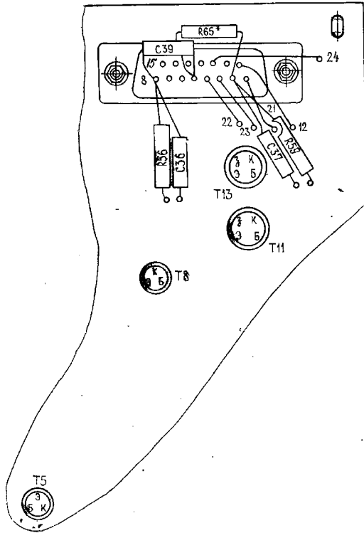
Рис. 10. Схема расположения элементов на усилителе Y (вид с обратной стороны).
