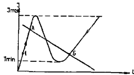
Рис. 2. Вольт-амперная характеристика туннельного диода.
