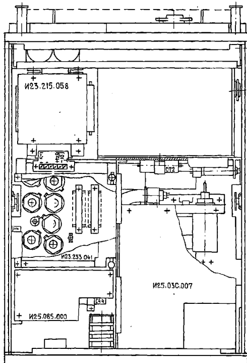
Рис. 4. Схема расположения установочных элементов и печатных плат (вид снизу).
