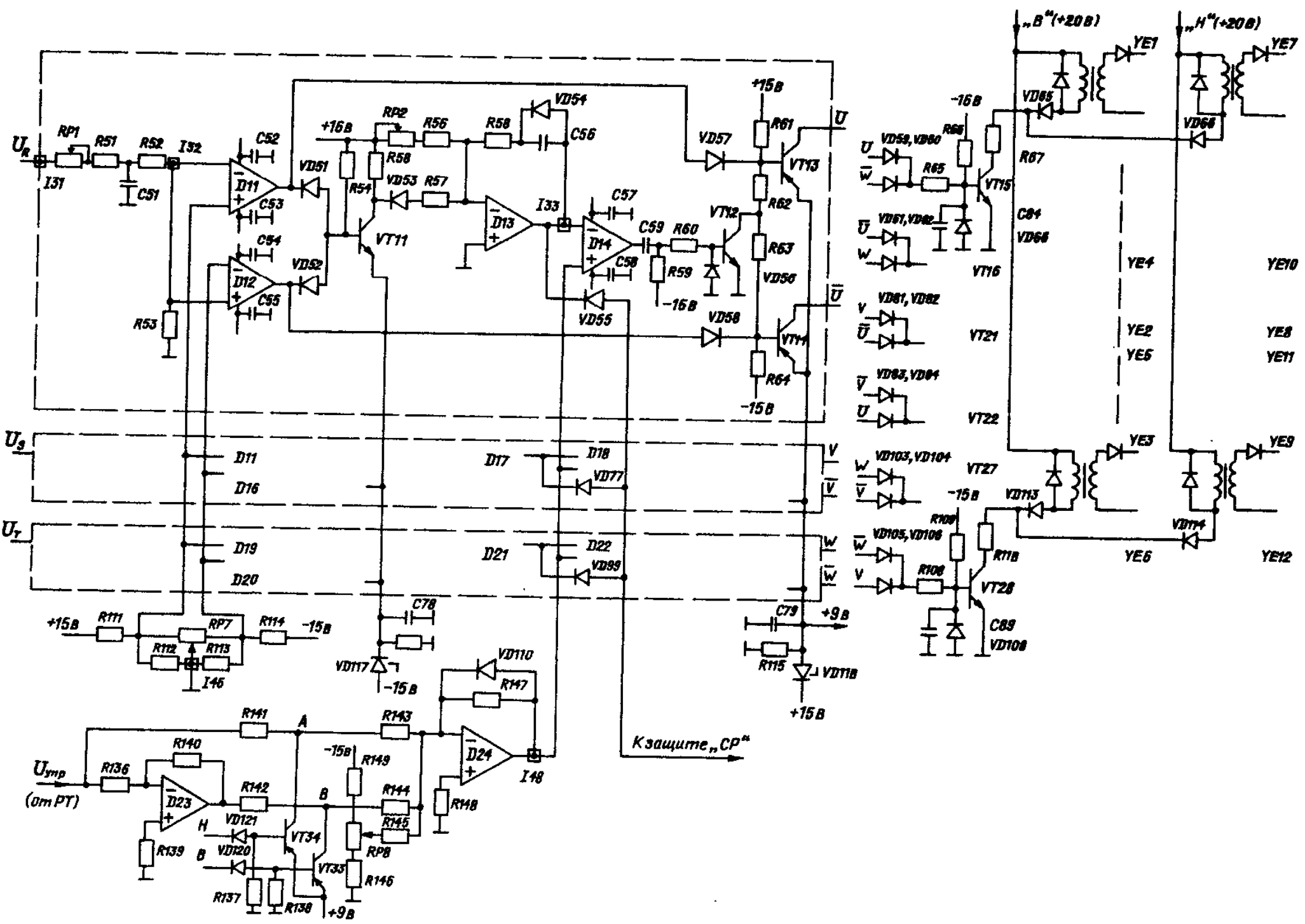
Рис. 4.14. Система импульсно-фазового управления
