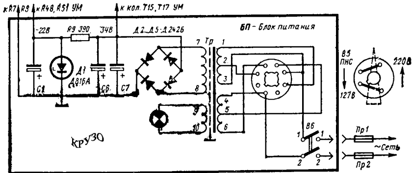
Принципиальная электрическая схема блока питания электрофона «Вега-101».
