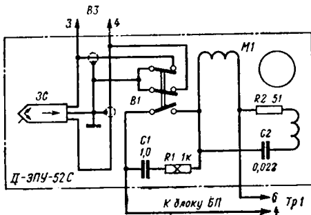
Принципиальная электрическая схема электропроигрывающего устройства электрофона «Вега-101».
