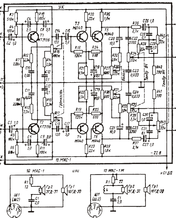
Принципиальная электрическая схема блока двухканального усилителя НЧ и громкоговорителя электрофона «Вега-101».
