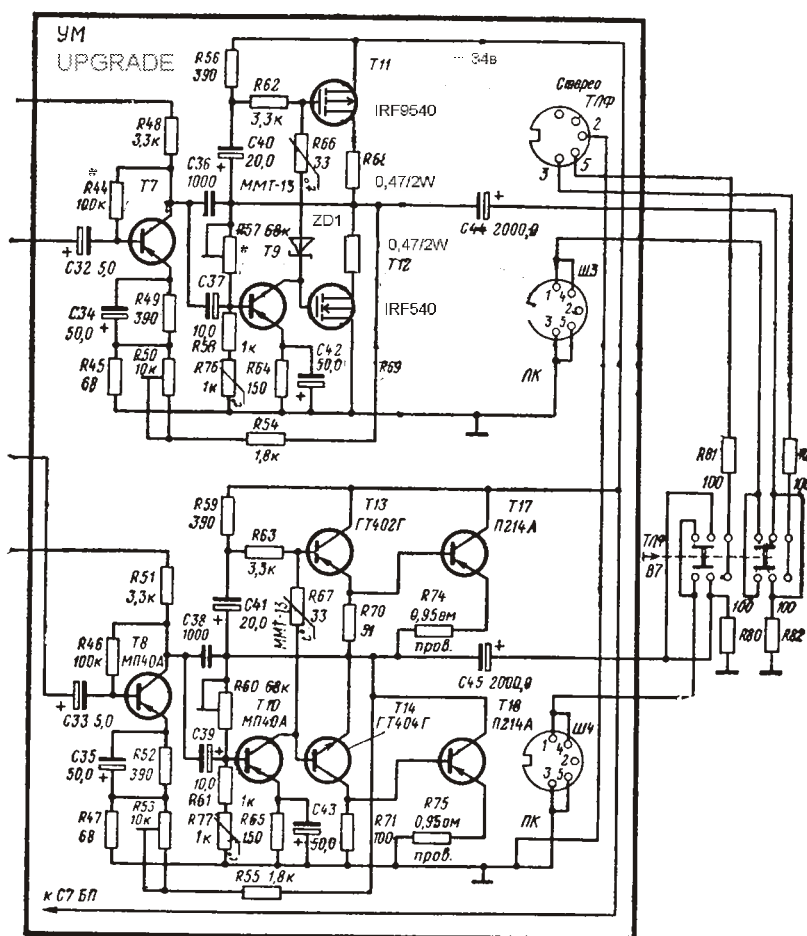
Принципиальная электрическая схема блока двухканального усилителя НЧ и громкоговорителя электрофона «Вега-101».
