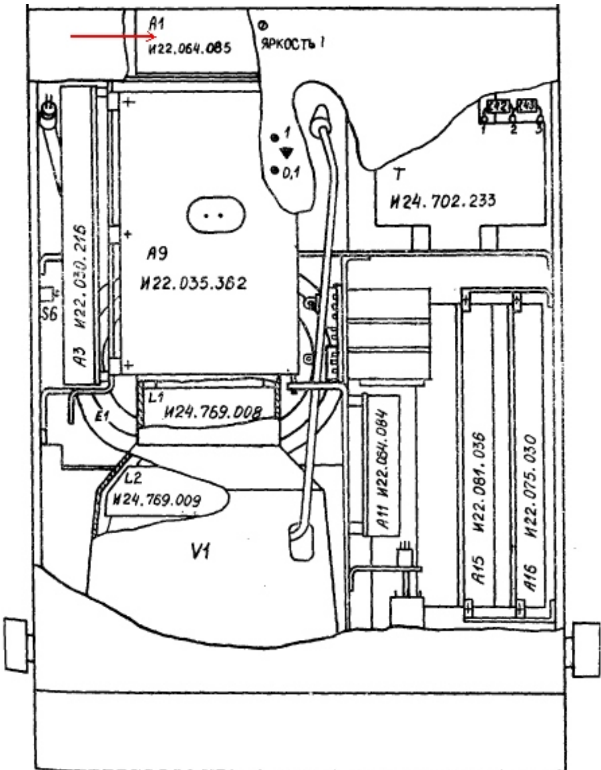
Рис. 3. Схема расположения установочных элементов и печатных плат в приборе С1-99 (вид сверху).
