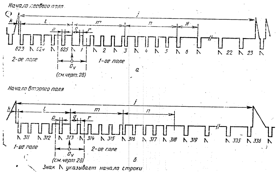
Гасящие, синхронизирующие и уравнивающие импульсы полей
