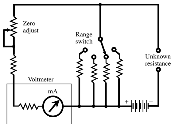
ohmmeter
