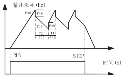
图 5-11 变频运行举例逻辑图
