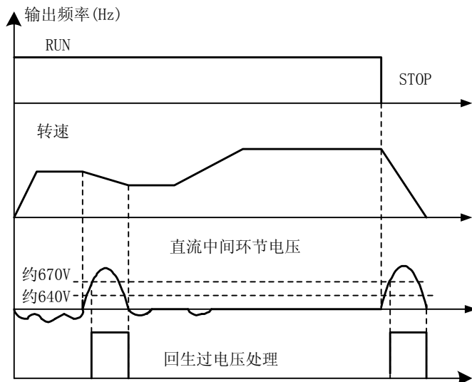
图 5-18 回升过电压处理
