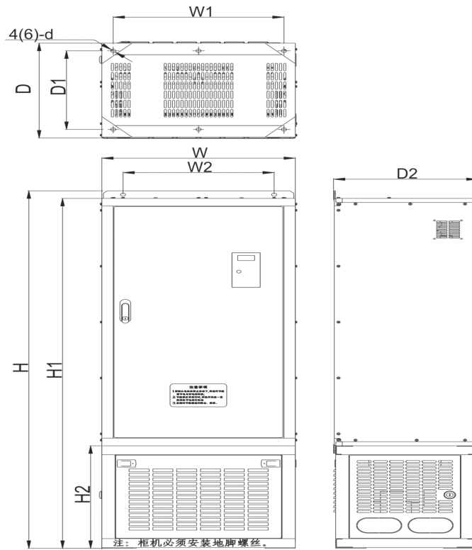
图 2-4 93kW 及以上带底座规格外形尺寸 表 2-4 93kW 及以上带底座外形尺寸和安装尺寸
