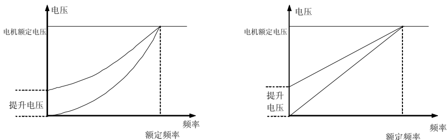
(a) 递减转矩曲线转矩提升示意图 (b) 恒转矩曲线转矩提升示意图
