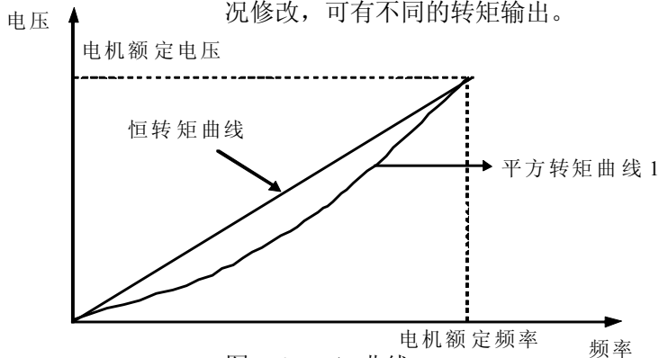
图 5-4 V/F 曲线
