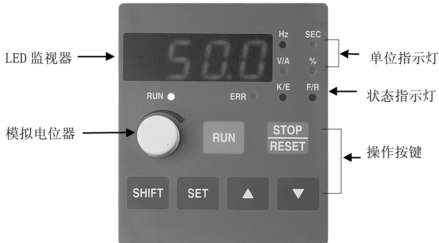
图 4-1 本机键盘各部分名称
