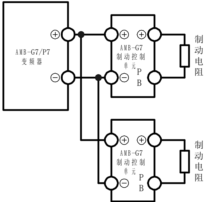
图 9-3 制动控制单元的并联安装
