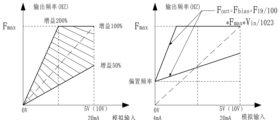
图 5-3a 模拟输入、频率增益与输出频率 图 5-3b 模拟输入、偏置频率与输出频率
