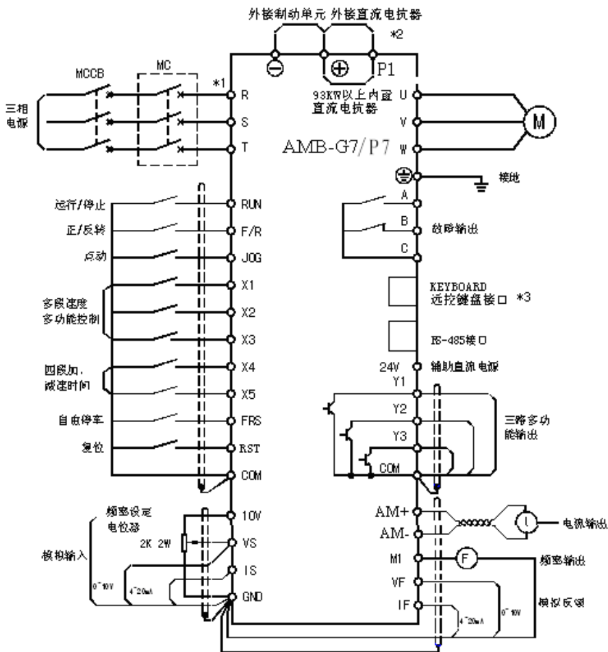
图 3-16 控制回路端子连接图
