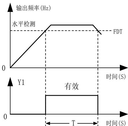
图 5-12 频率水平检测
