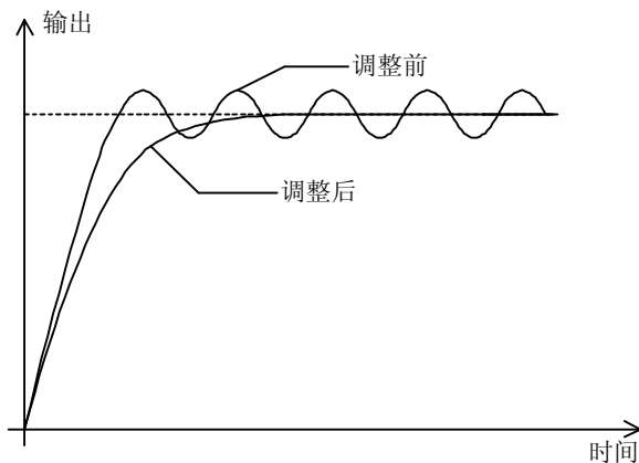
图 5-21 抑制输出周期振荡
