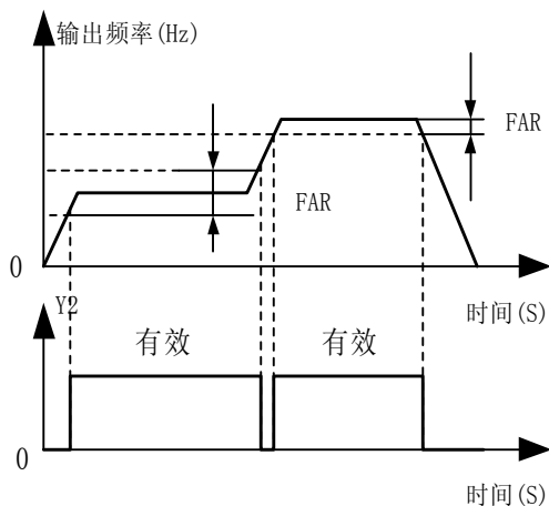
图 5-13 频率等效范围检测
