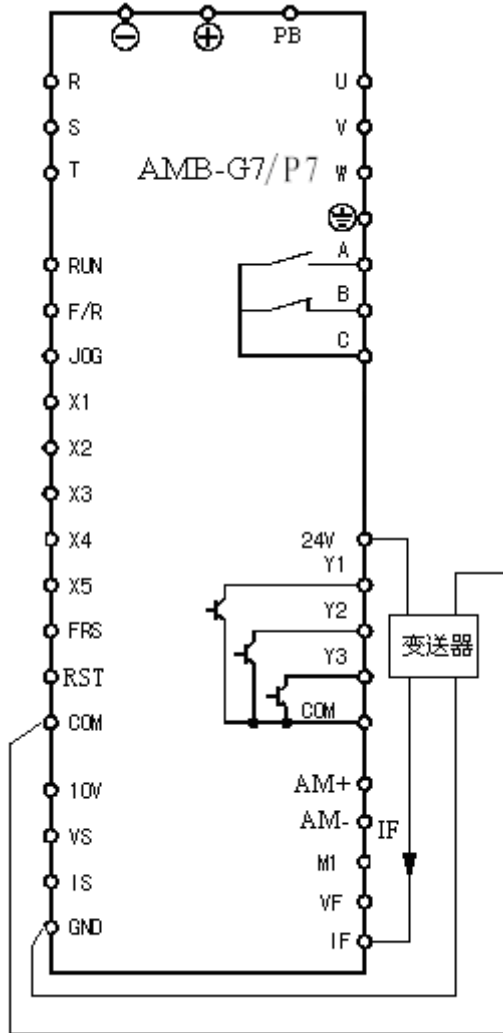
图 5-23 电流型反馈检测接线
