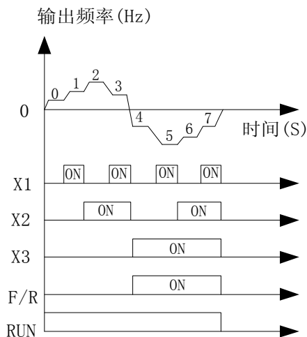
图 5-8 多段速度运行逻辑图
