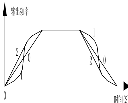
图 5-14 加速/减速模式
