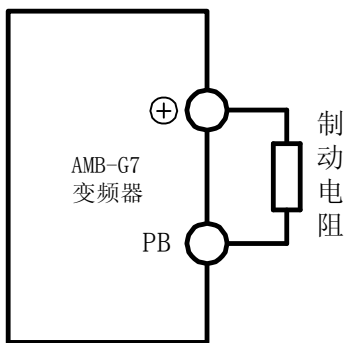
图 9-1 制动电阻的安装
