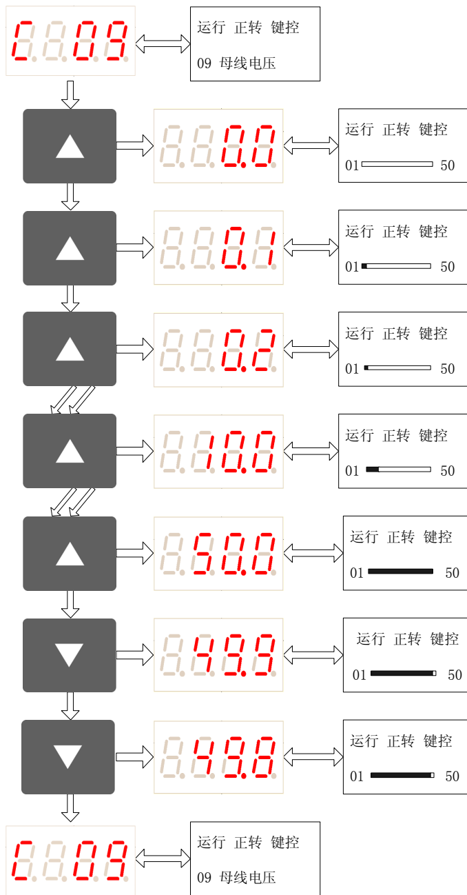
图 4-9 键盘数字电位器操作流程
