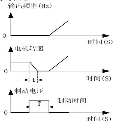
图 5-7 启动直流制动过程
