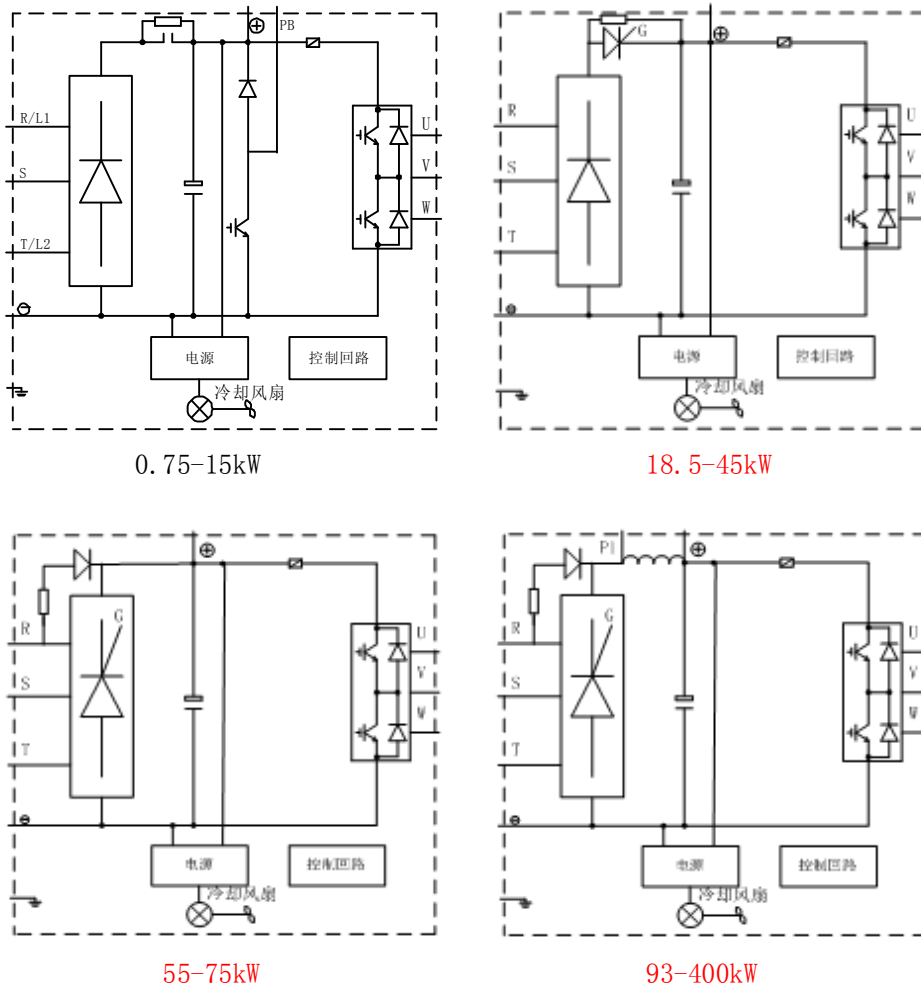
图 3-5 变频器主电路组成
