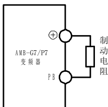
图 3-14 制动电阻的安装
