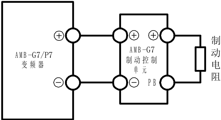
图 9-2 制动控制单元的安装
