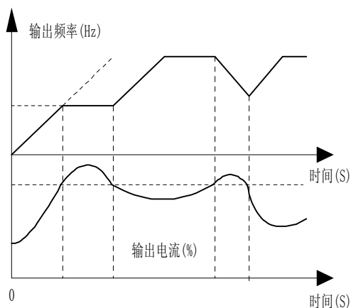
图 5-17 电流限幅动作过程
