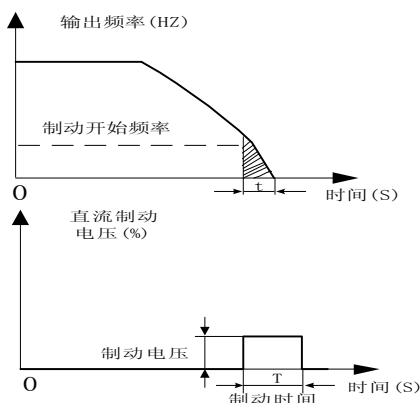
图 5-6 停车减速直流制动过程
