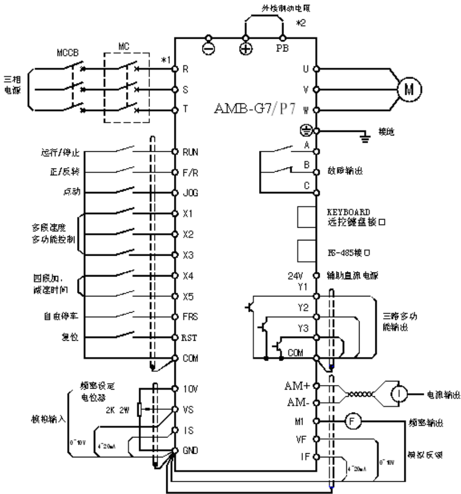
图 3-2 15kW 及以下规格 G7/P7 变频器连接图
