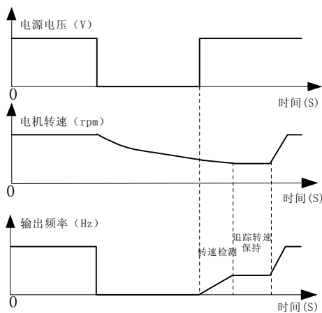
图 5-16 转速追踪示意图
