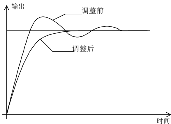
图 5-20 抑制输出超调
