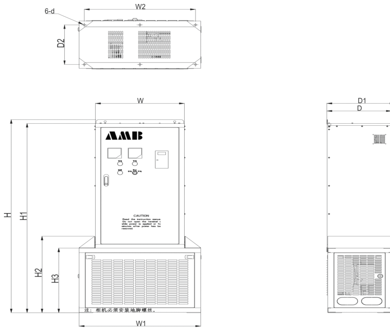
图 2-5 93kW 及以上带配电柜规格外形尺寸 表 2-5 93kW 及以上带配电柜外形尺寸和安装尺寸
