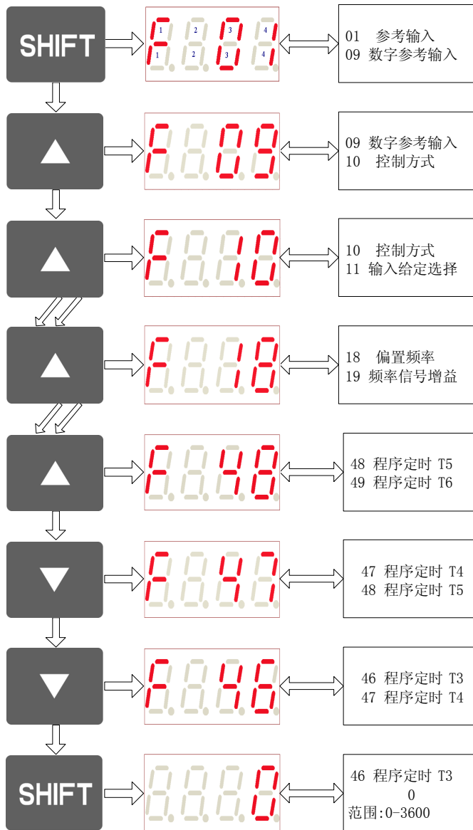
图 4-4 功能代码查询操作流程
