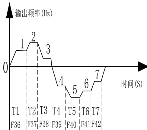
图 5-9 程序运行逻辑图
