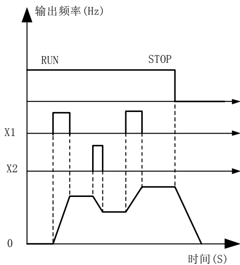
图 5-15a 步进方式 1
