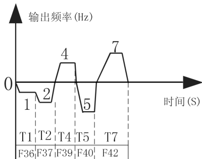
图 5-10 程序运行举例逻辑图
