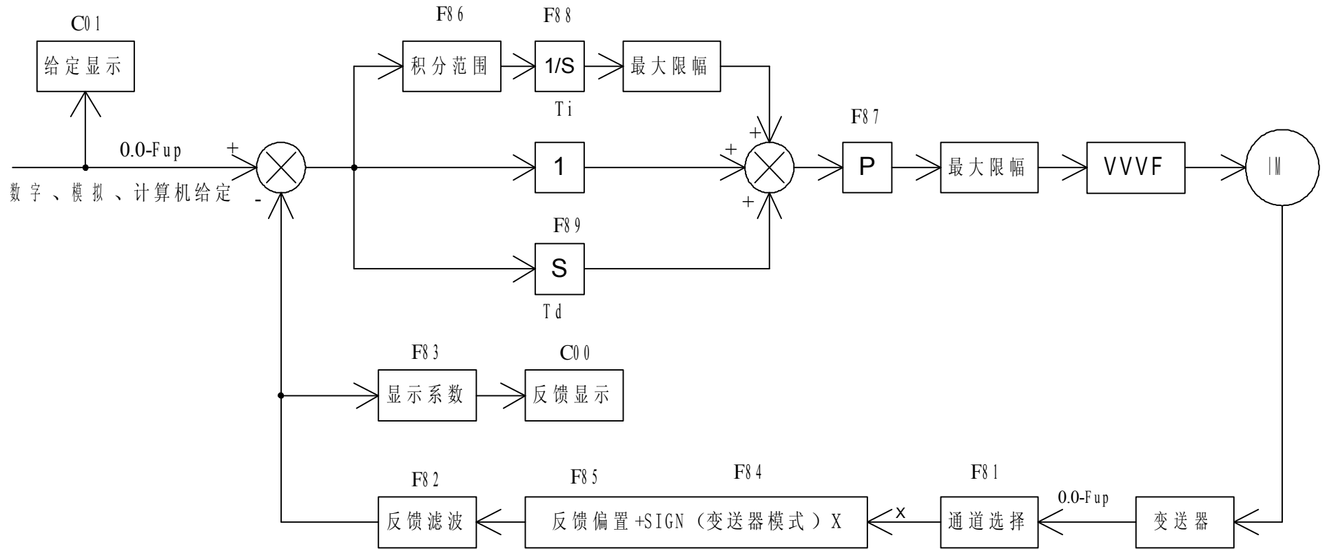
图 5-19 PID 闭环控制框图
