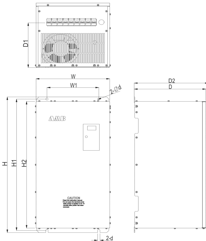
图 2-2 75Kw 及以下规格外形尺寸 表 2-2 75Kw 及以下外形尺寸和安装尺寸
