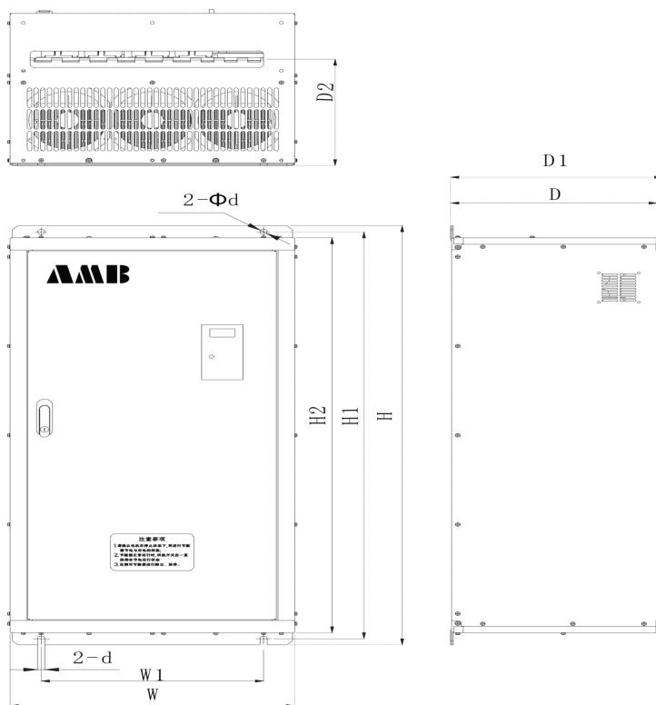
图 2-3 93kW 及以上挂机规格外形尺寸 表 2-3 93kW 及以上挂机外形尺寸和安装尺寸
