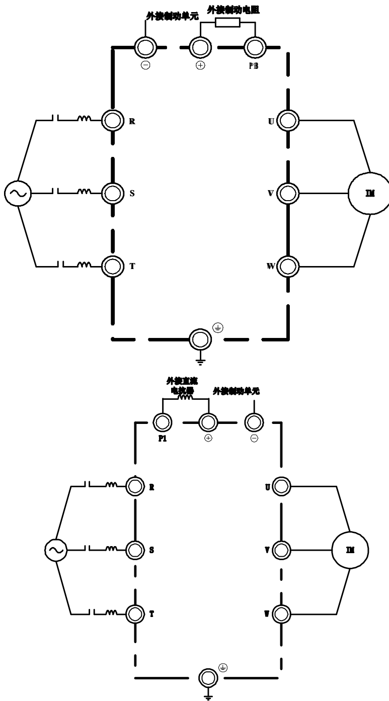
图 3-6 变频器主电路标准接线
