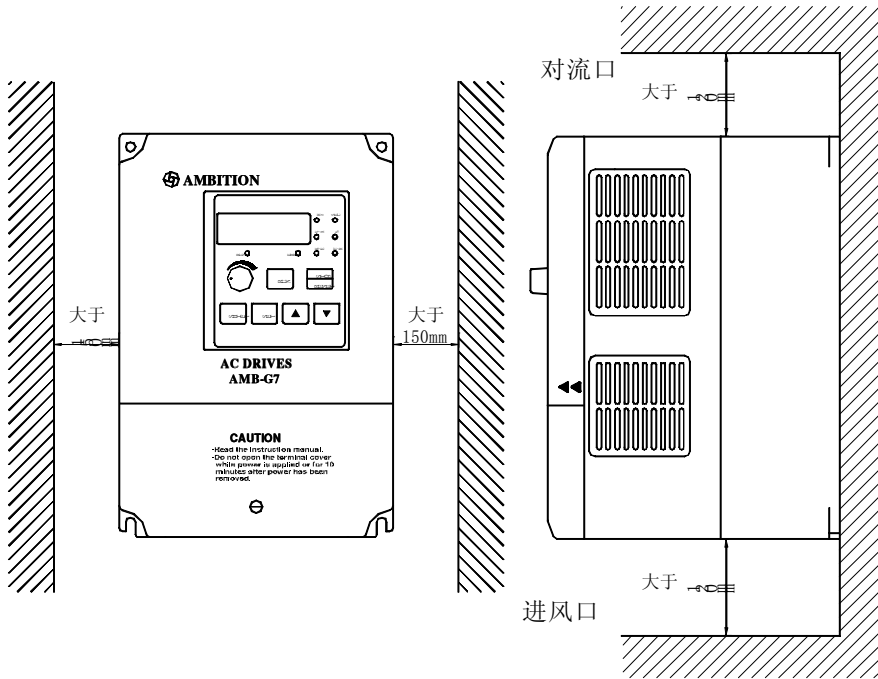
图 2-6 G7/P7 变频器安装方向和空间
