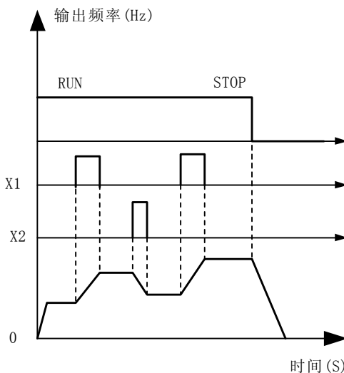
图 5-15b 步进方式 2
