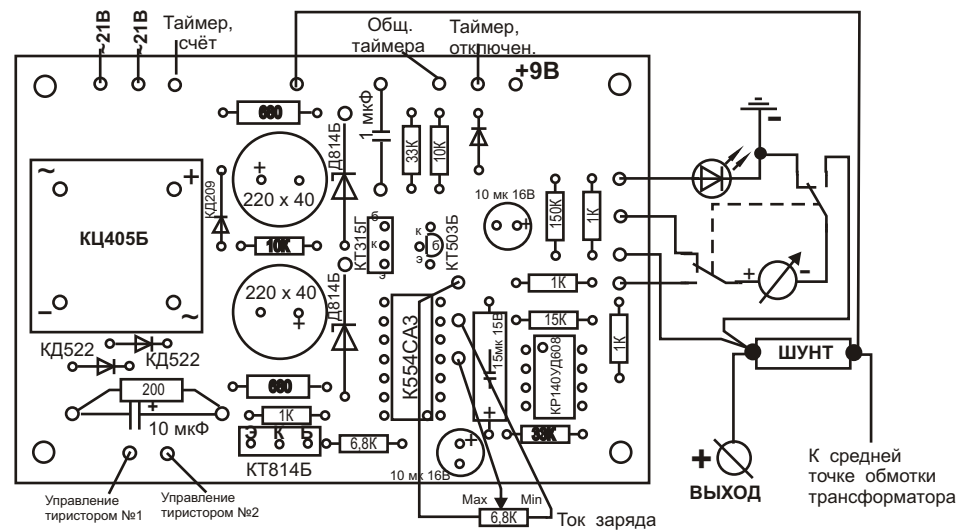
Схема автоматического блока зарядки автомобильных аккумуляторов
