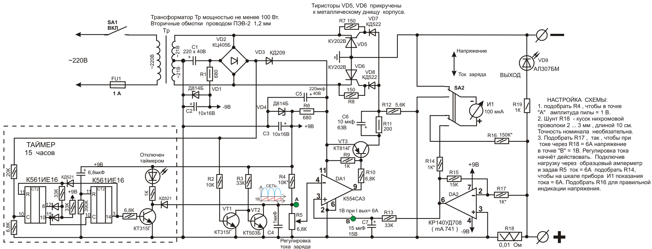
Схема автоматического блока зарядки автомобильных аккумуляторов
